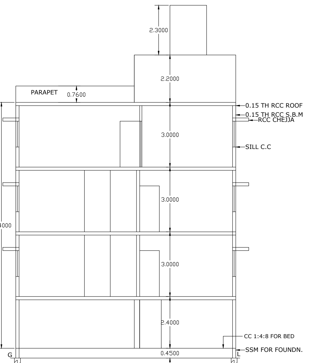
SECTION A-A
